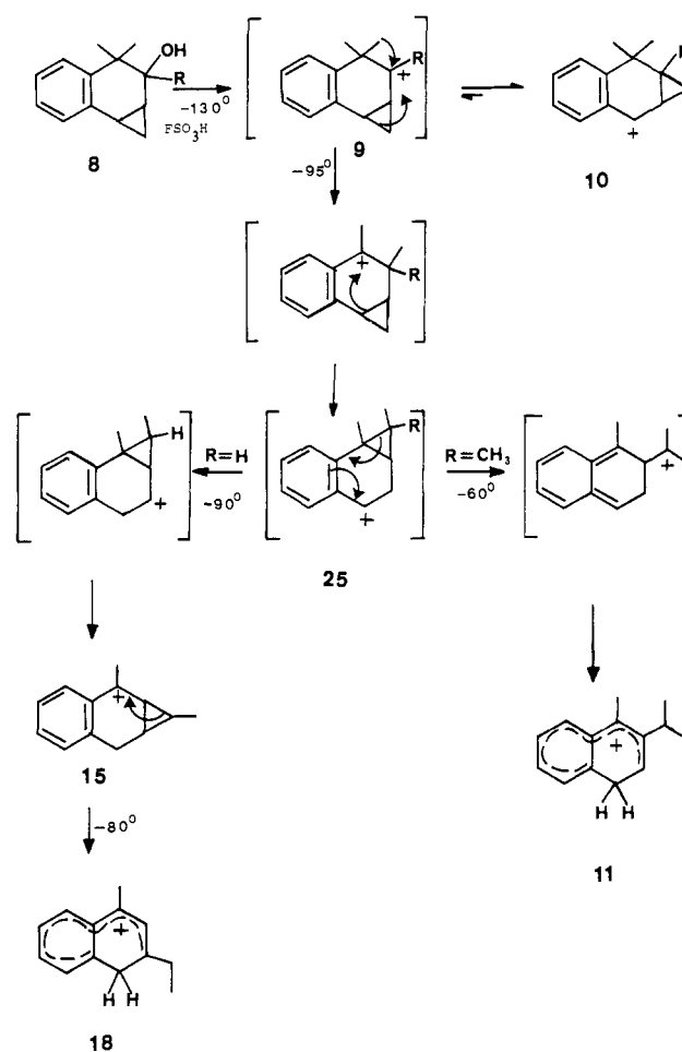
Scheme VI
